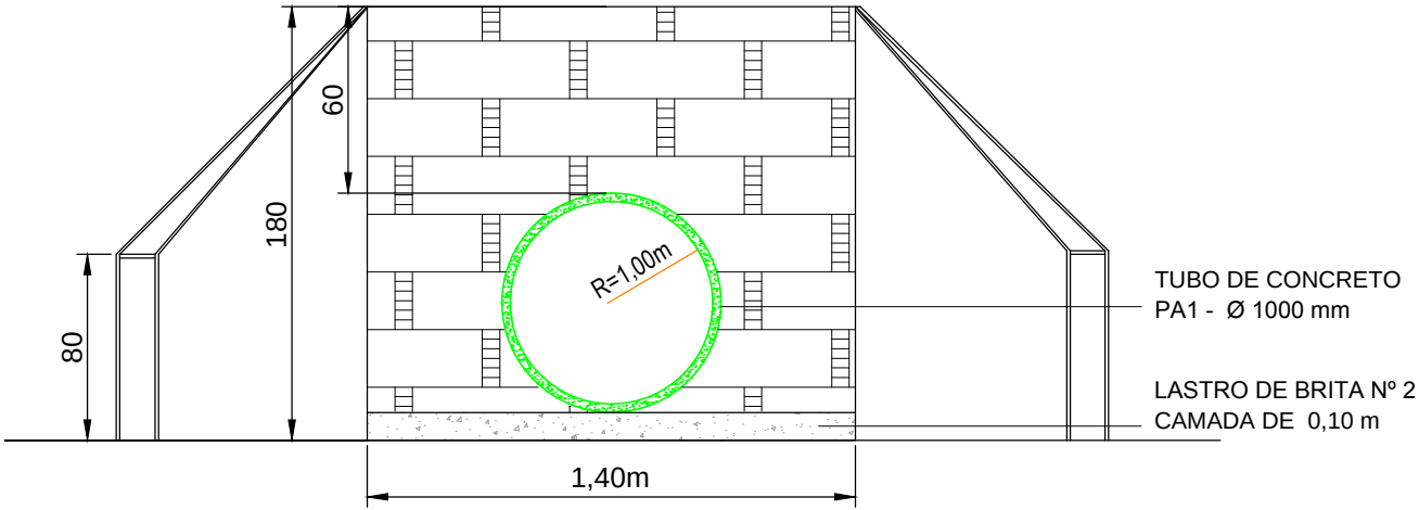
CORTE - ALAS (Montante) SEM ESCALA
