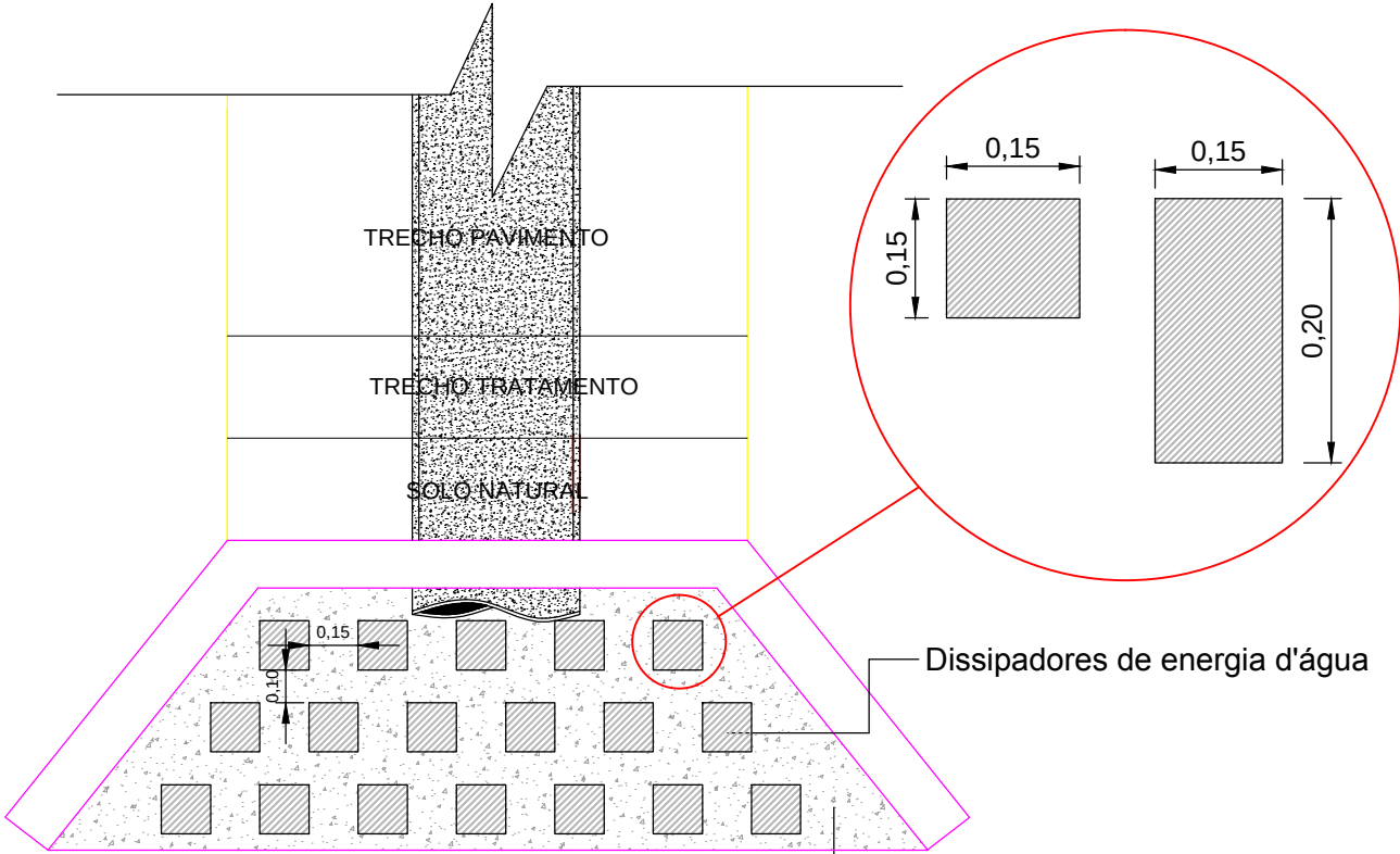
PLANTA BAIXA - ALAS (Detalhe Jusante) SEM ESCALA
