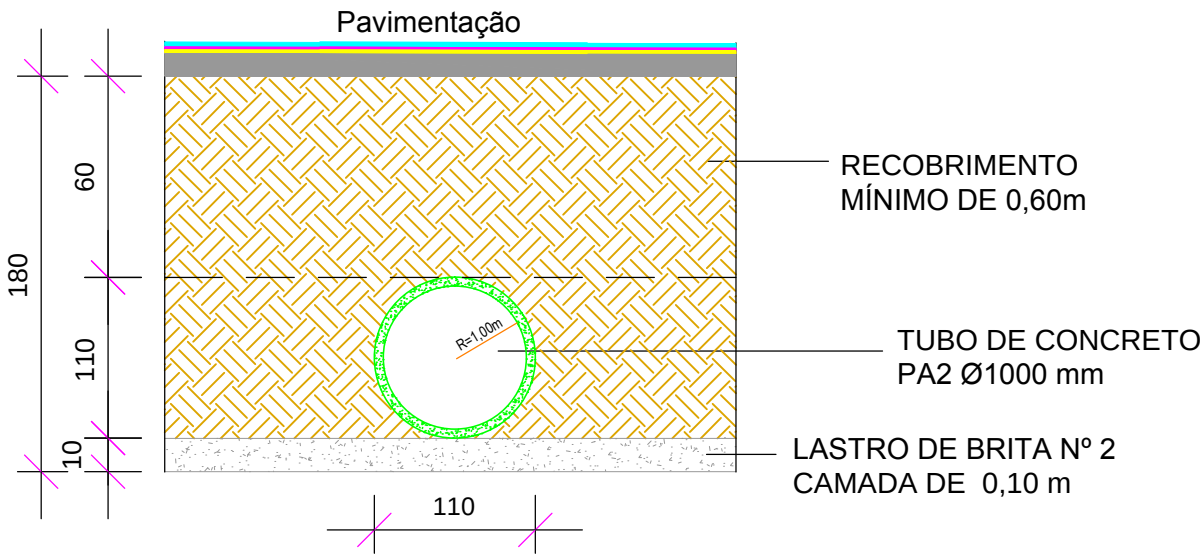
DETALHE ASSENTAMENTO TUBOS SEM ESCALA
