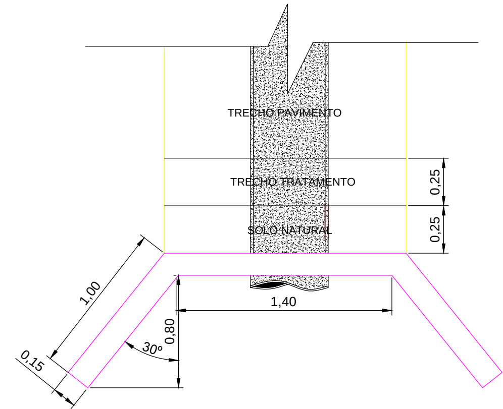
PLANTA BAIXA - ALAS (Detalhe Montante) SEM ESCALA
