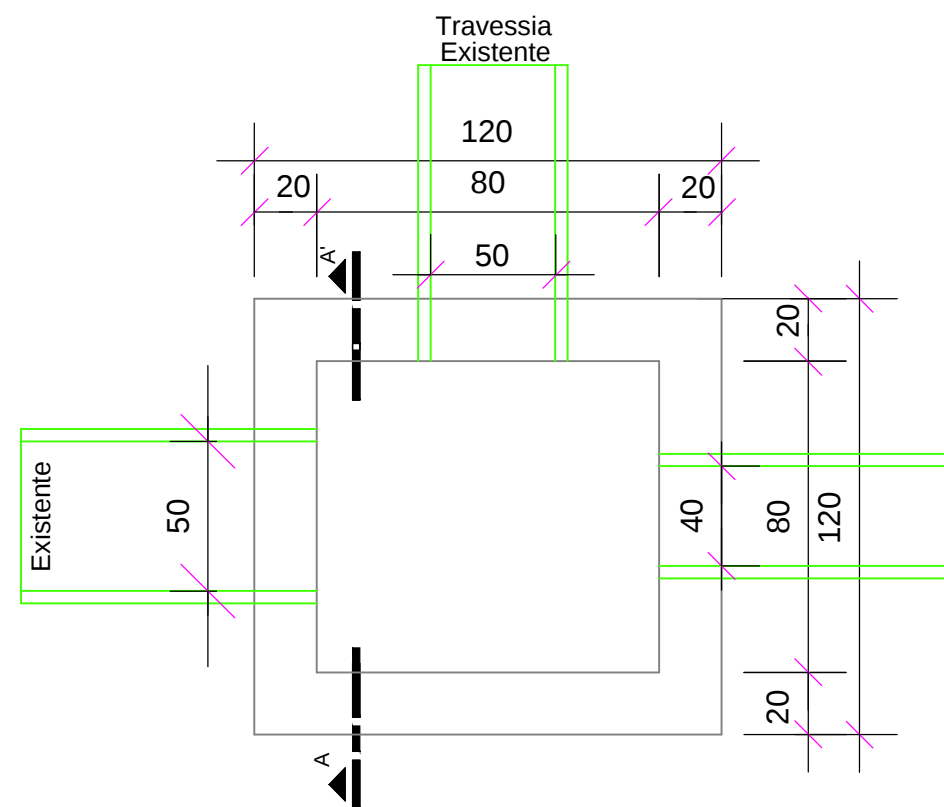
PLANTA BAIXA - POÇO DE VISITA 0,80 x 0,80m (interno) SEM ESCALA
