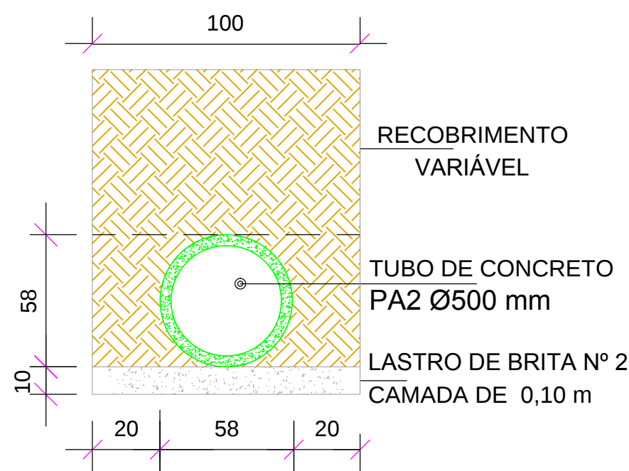
SEÇÃO TIPO DA TUBULAÇÃO PA2 Ø 500 mm SEM ESCALA
