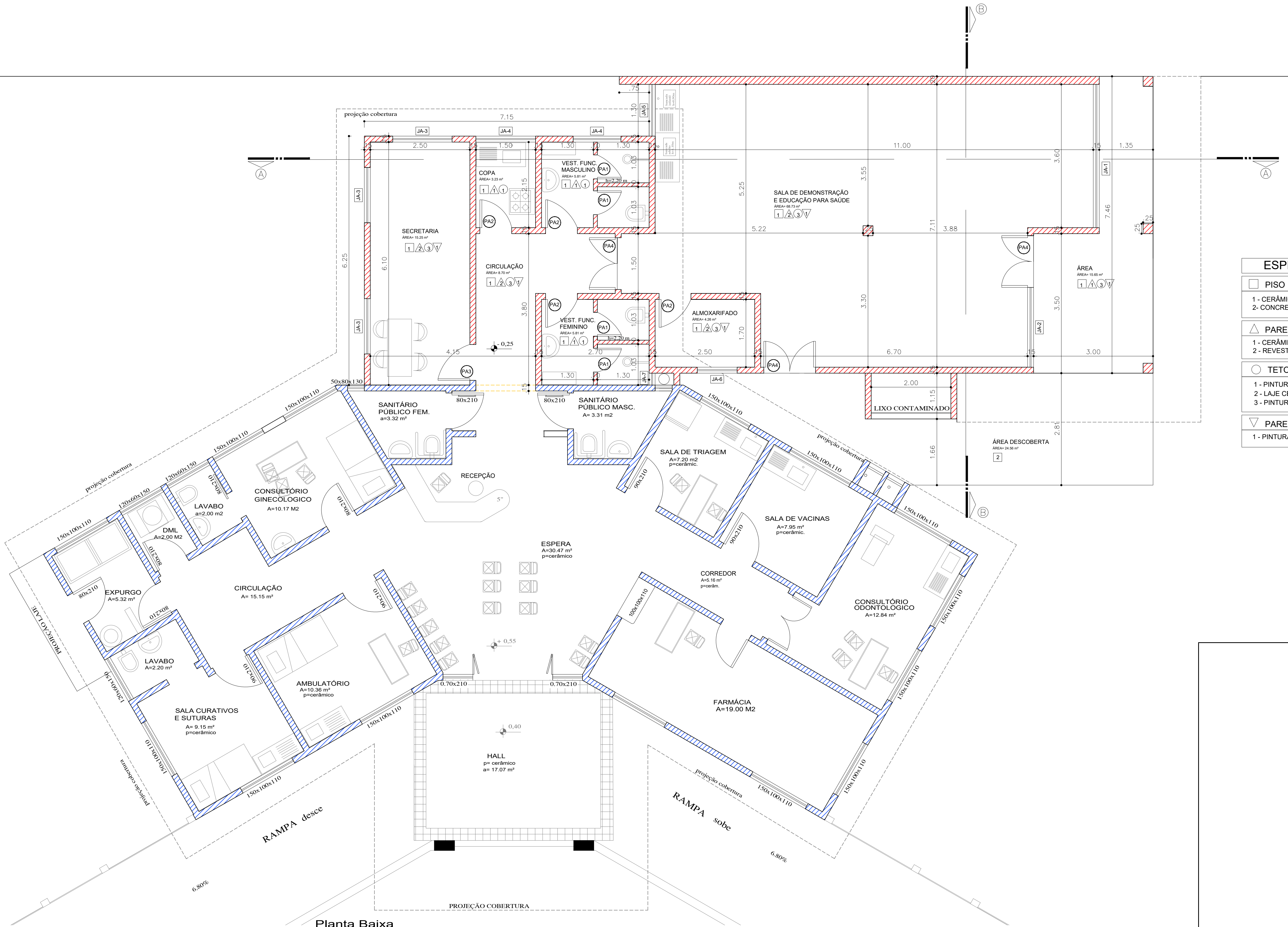
Planta Baixa Escala 1: 50 Área à Existente: 187,01 m² Área à Construir: 141,86 m²
