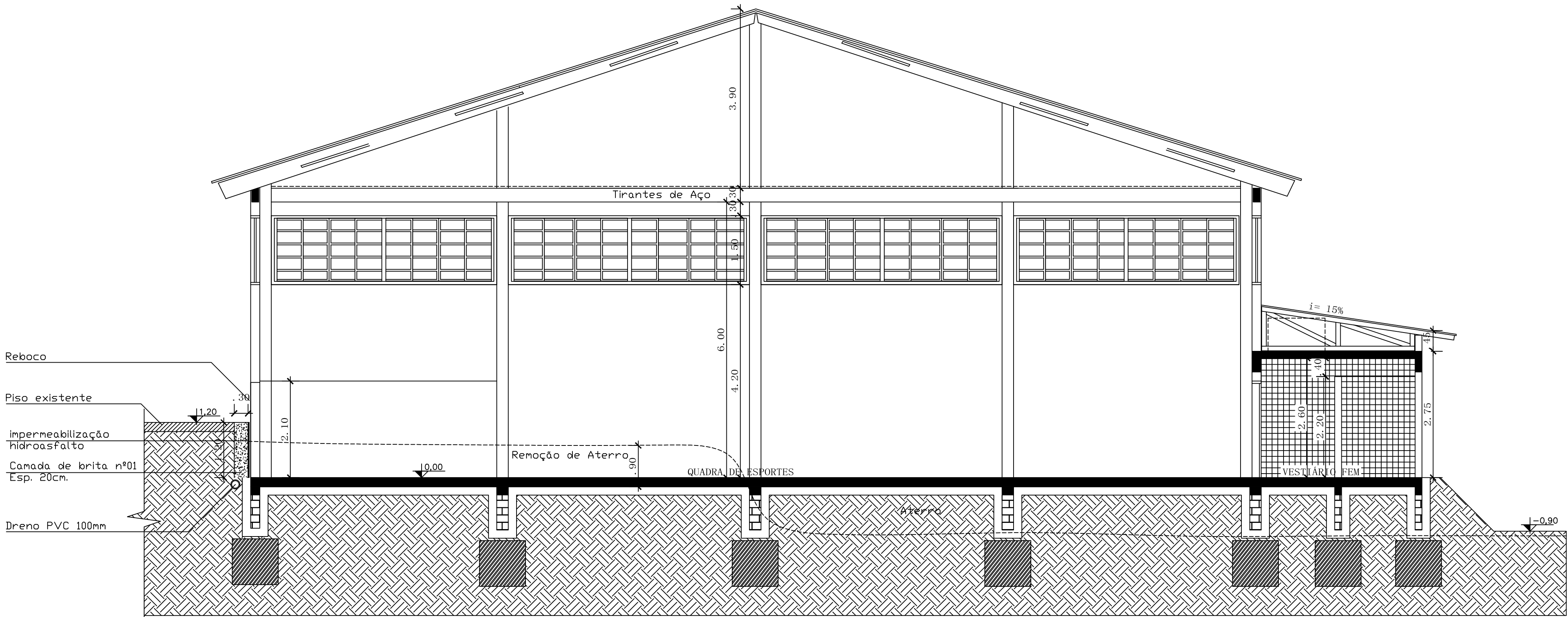
CORTE BB
