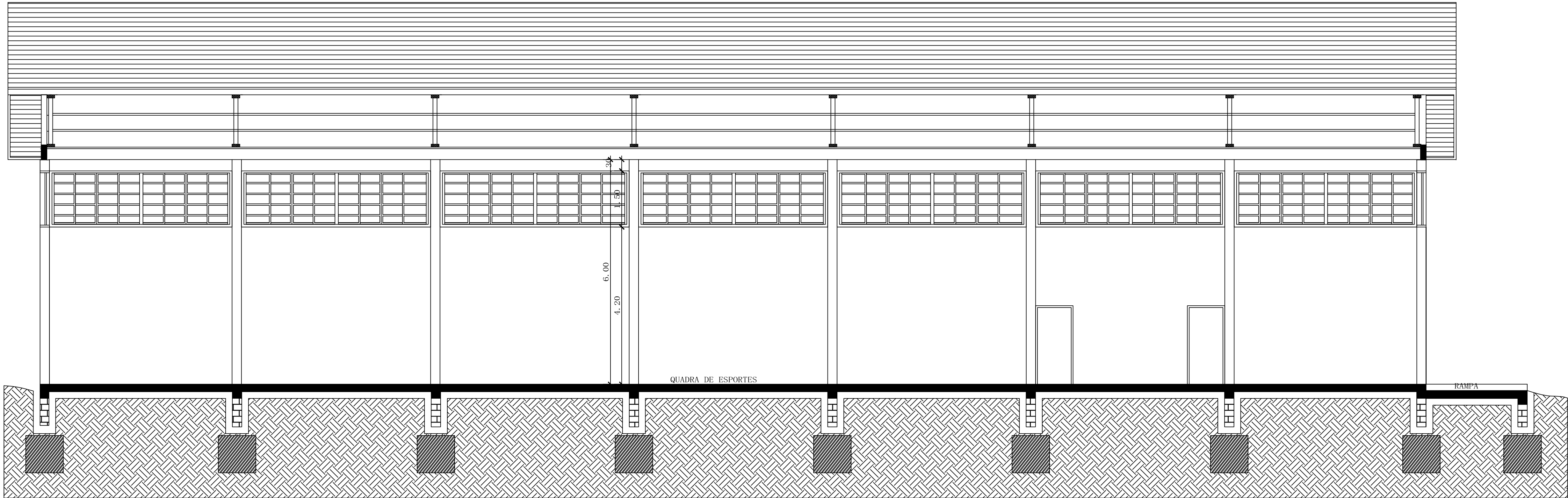
CORTE AA
