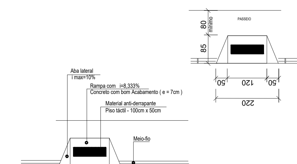
DETALHE RAMPA DE ACESSO A CADEIRANTES SEM ESCALA
