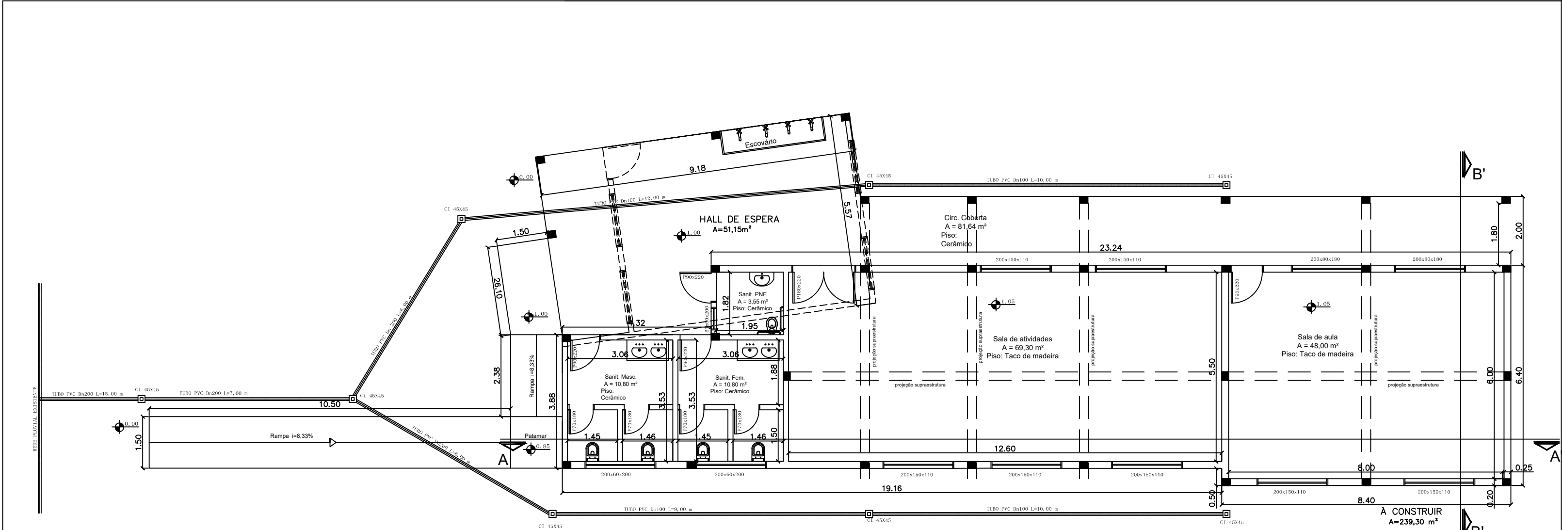
PLANTA BAIXA
