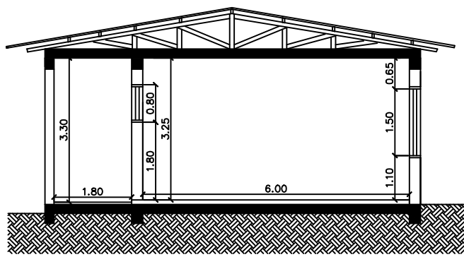
CORTE BB'
