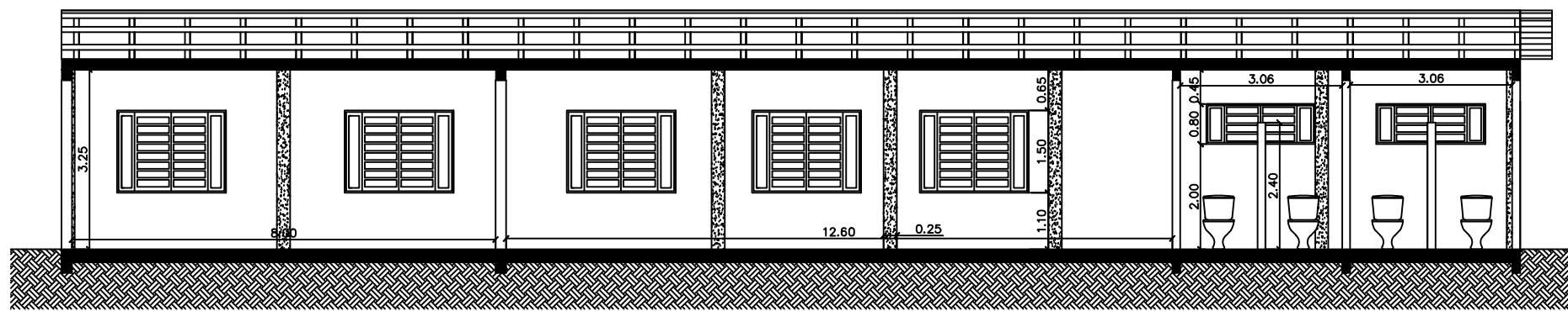
CORTE AA'
