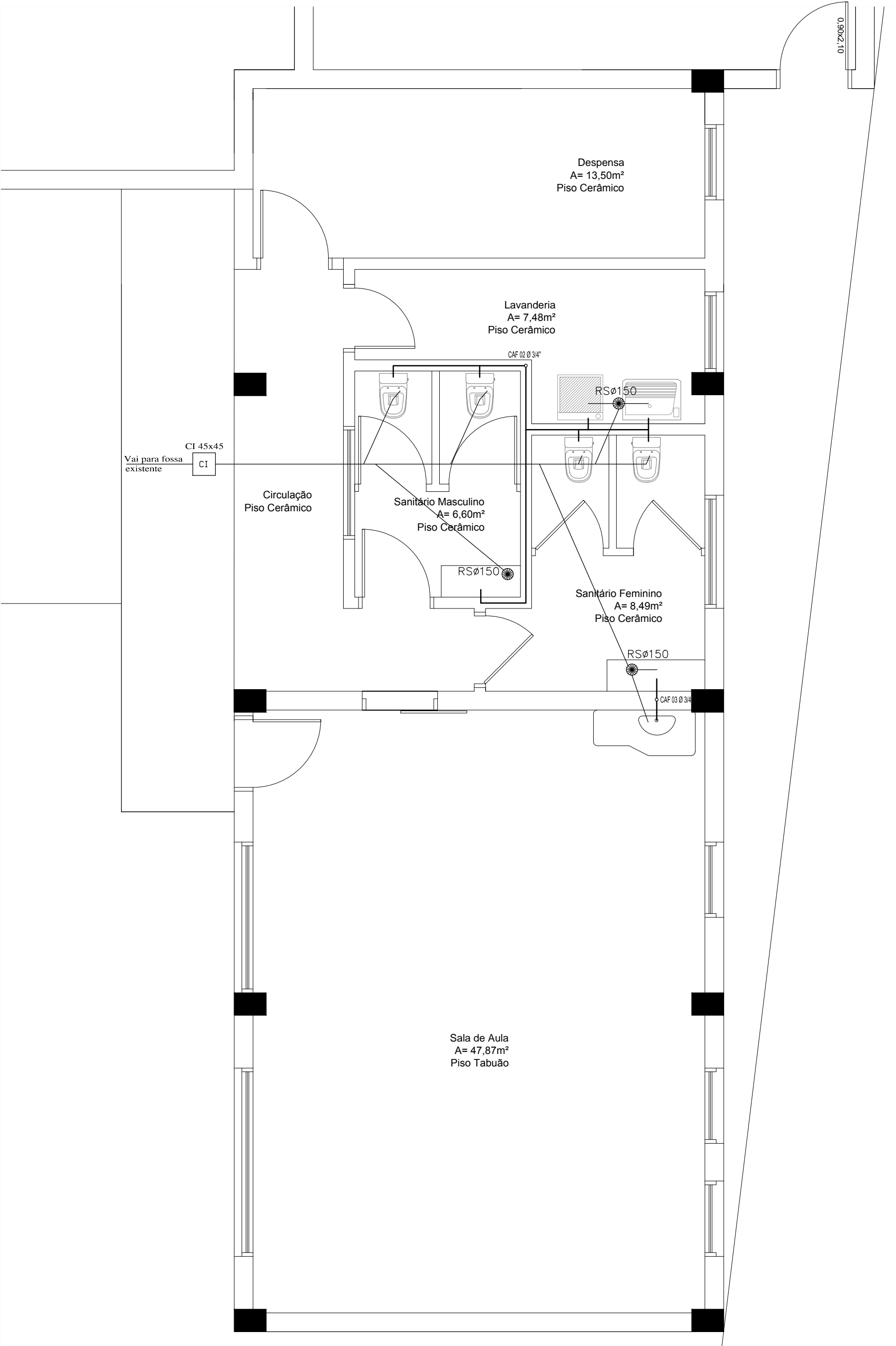
PLANTA BAIXA SALA E SANITÁRIOS
