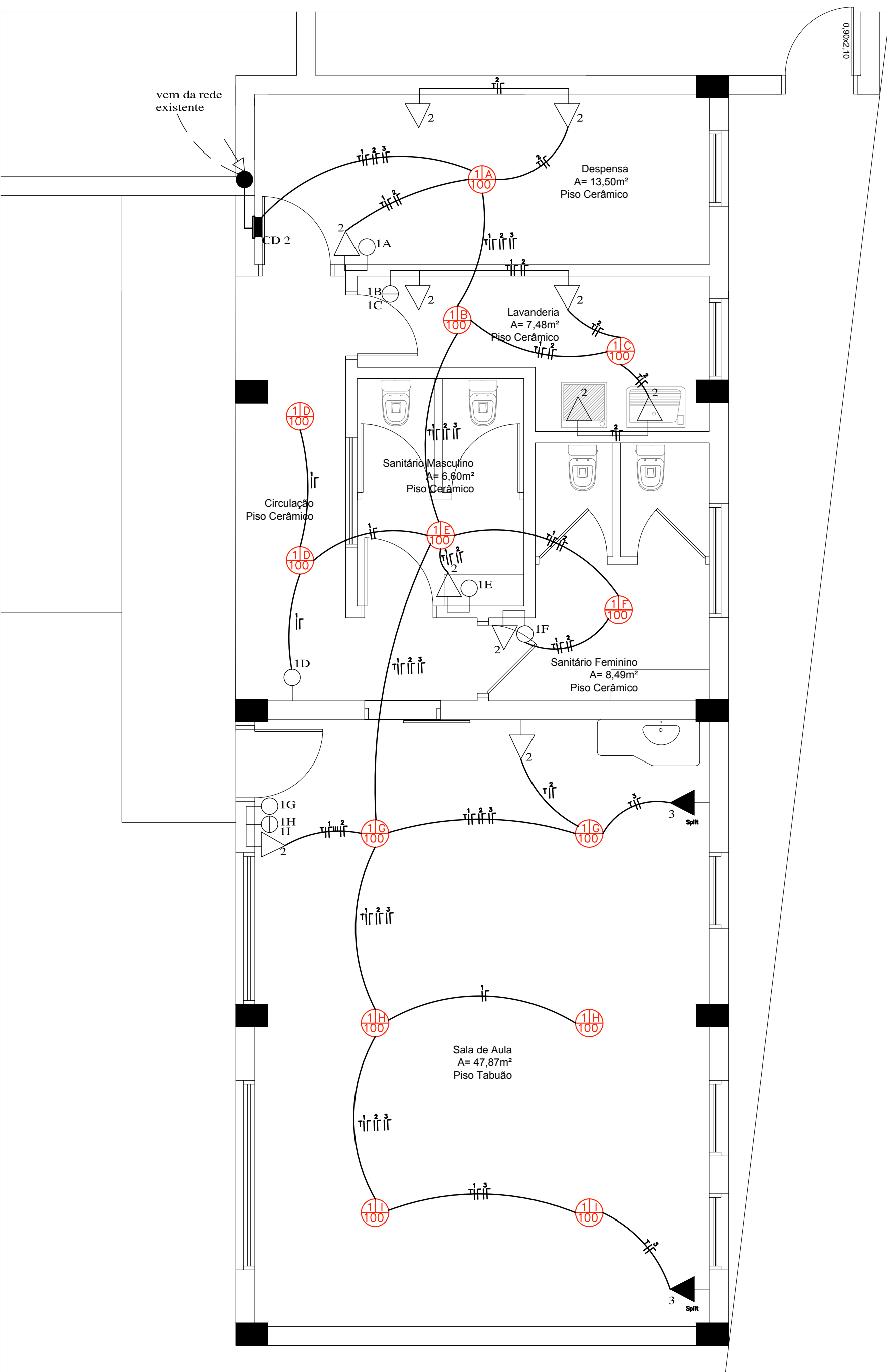
PLANTA BAIXA SALA E SANITÁRIOS
