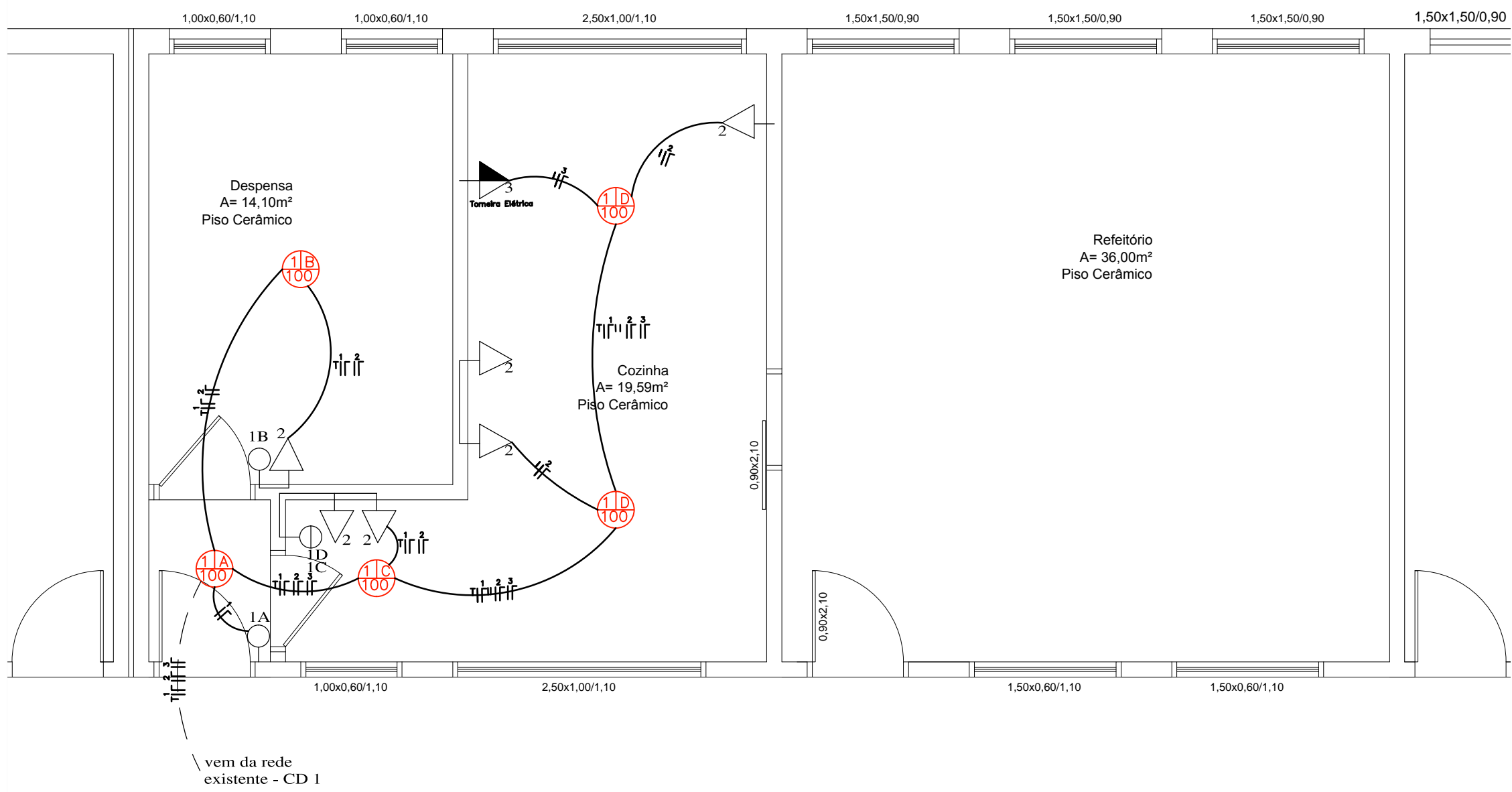
ELÉTRICO COZINHA E REFEITÓRIO
