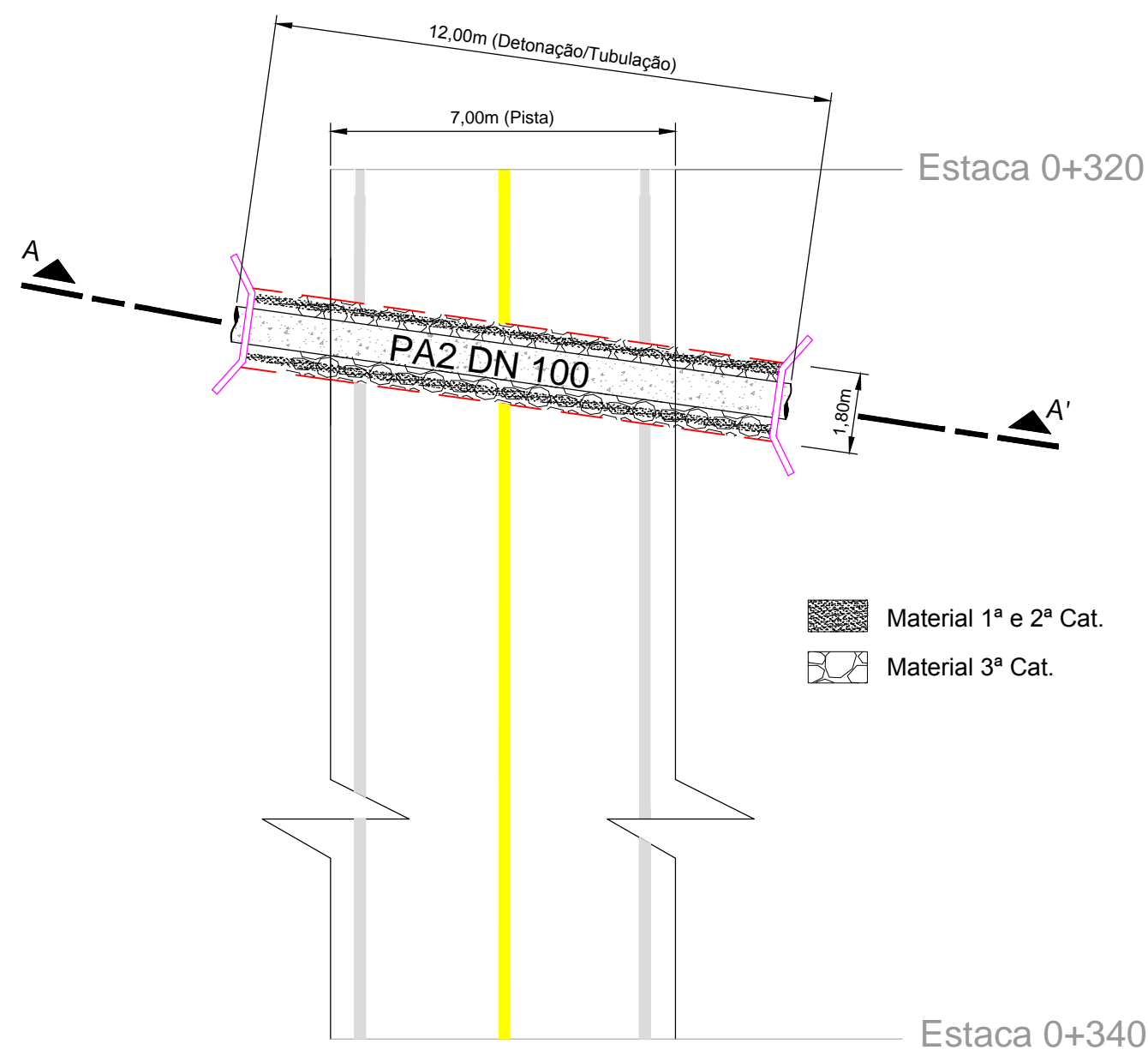
PLANTA BAIXA - MATERIAL DE 3ª CAT. SEM ESCALA
