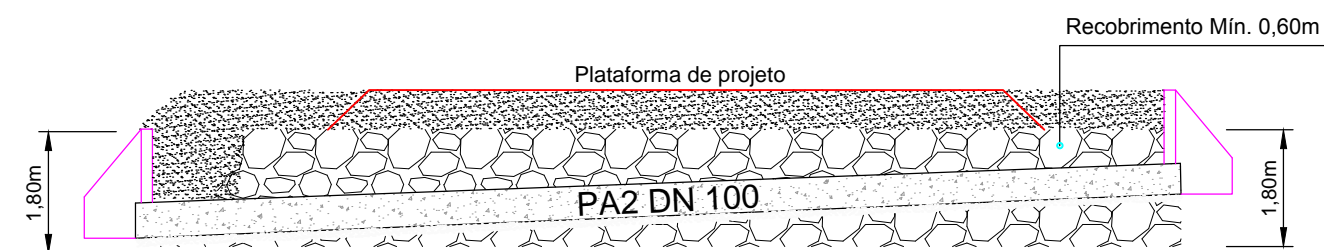
CORTE AA'- MATERIAL DE 3ª CAT. SEM ESCALA
