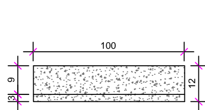
DETALHE DO MEIO-FIO - MFC 05
