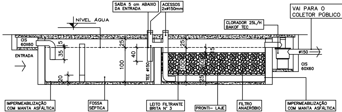
CORTE C/C FOSSA SÉPTICA E FILTRO ANAERÓBIO ESCALA 1/50
