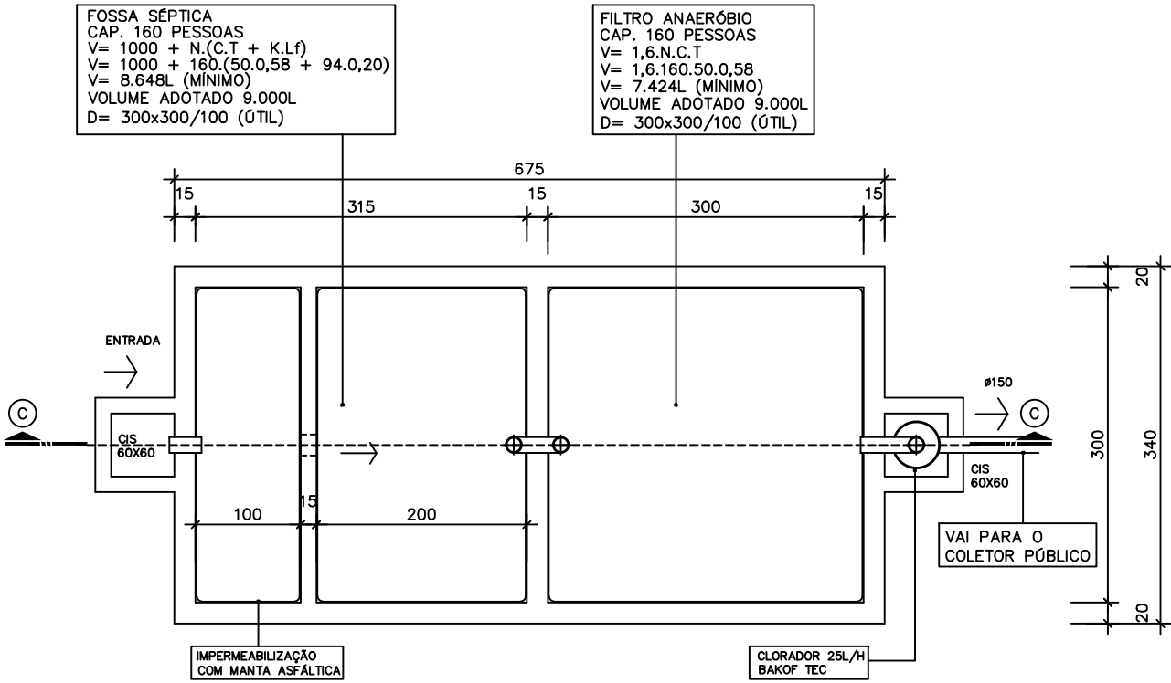
PLANTA BAIXA FOSSA SÉPTICA E FILTRO ANAERÓBIO ESCALA 1/50
