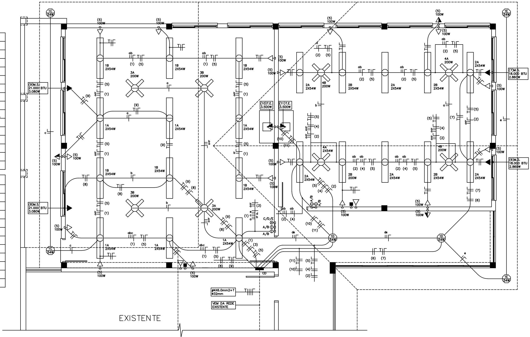
PROJETO ELÉTRICO ESCALA 1/50
