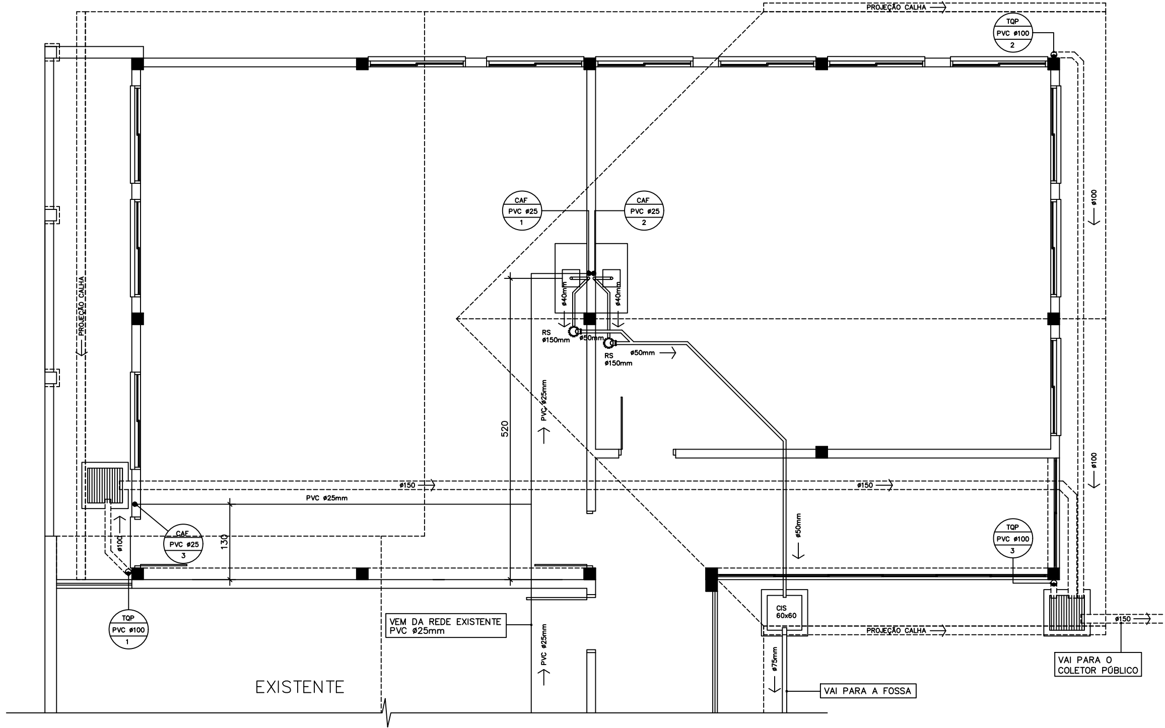
PLANTA BAIXA PROJETO HIDROSSANITÁRIO E PLUVIAL ESCALA 1/50
