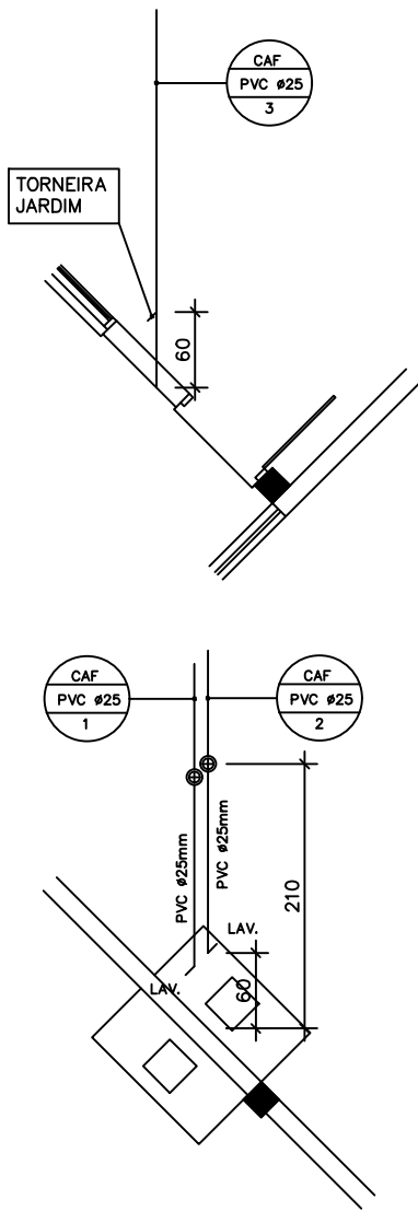
ESTEREOGRAMAS ESCALA 1/50
