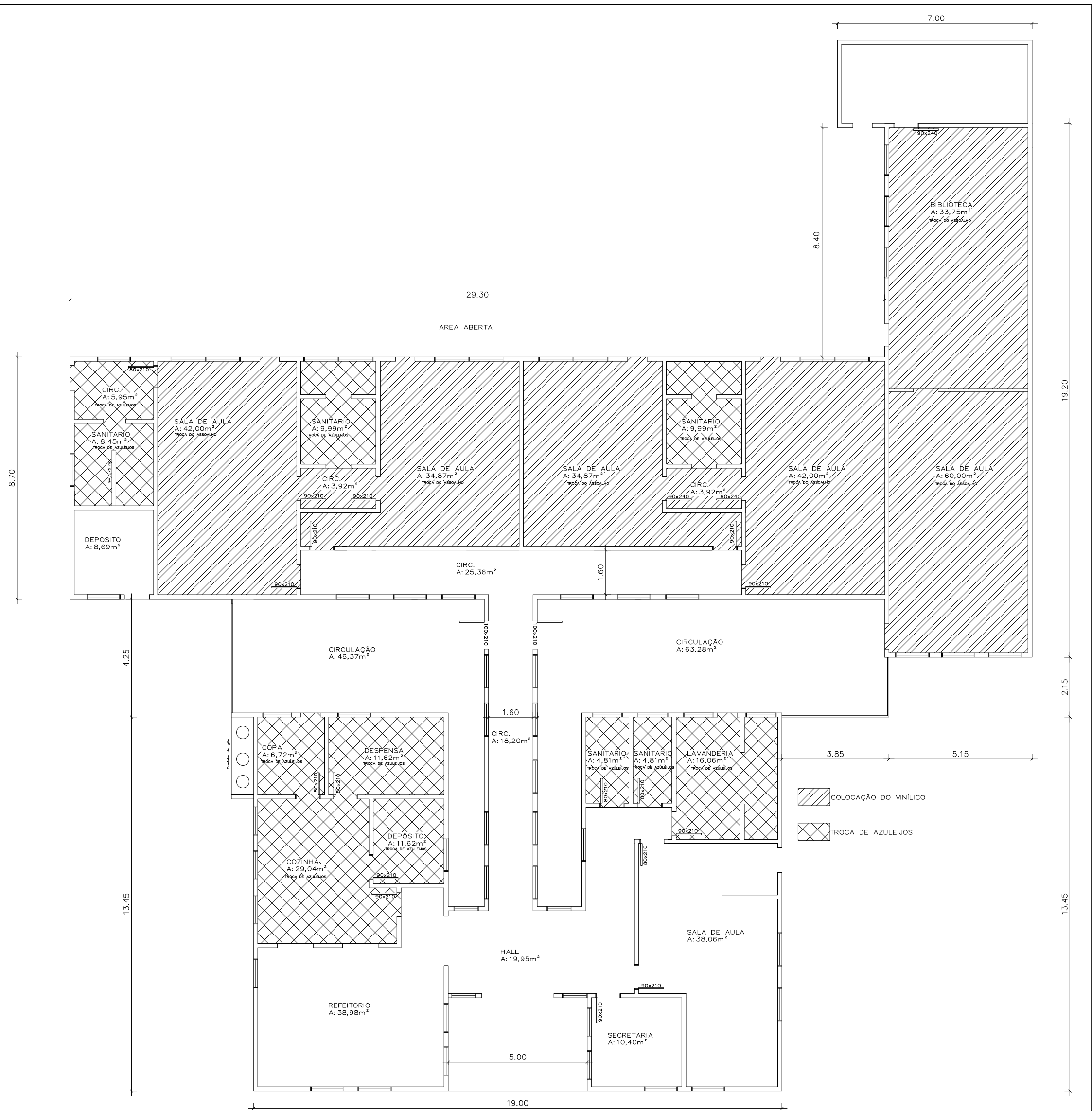
PLANTA BAIXA TÉRREO A. 735,00m2
